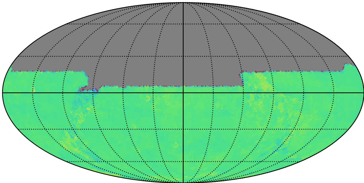
too_ignore_100_1v3.4_10yrs u: Kuiper rotTelPos
