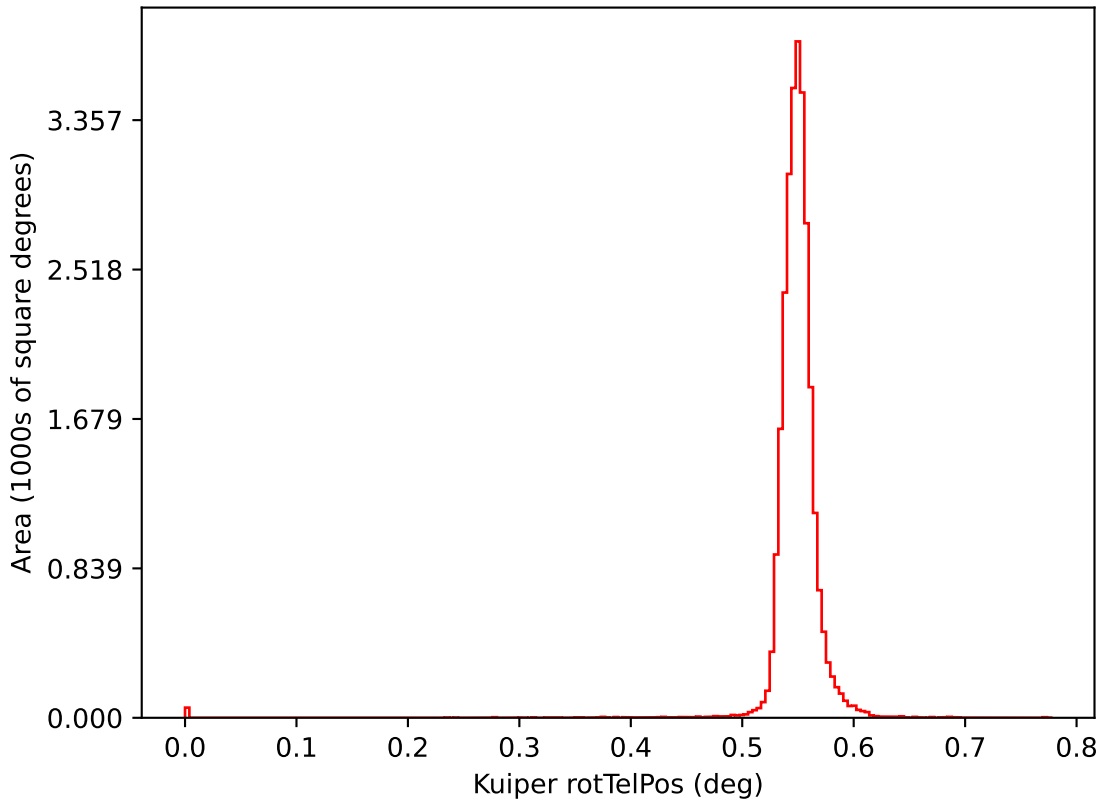
too_ignore_100_1v3.4_10yrs i: Kuiper rotTelPos
