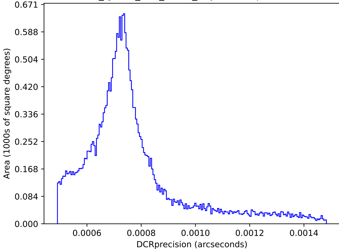
too_ignore_100_1v3.4_10yrs : DCRprecision
