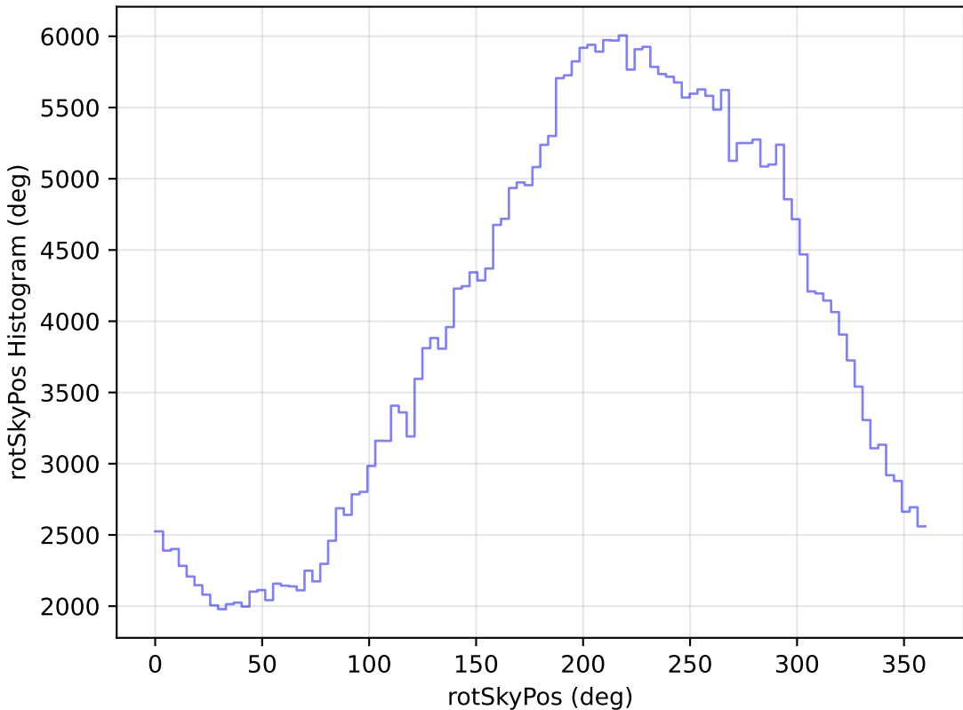
too_ignore_100_1v3.4_10yrs WFD y band: rotSkyPos Histogram
