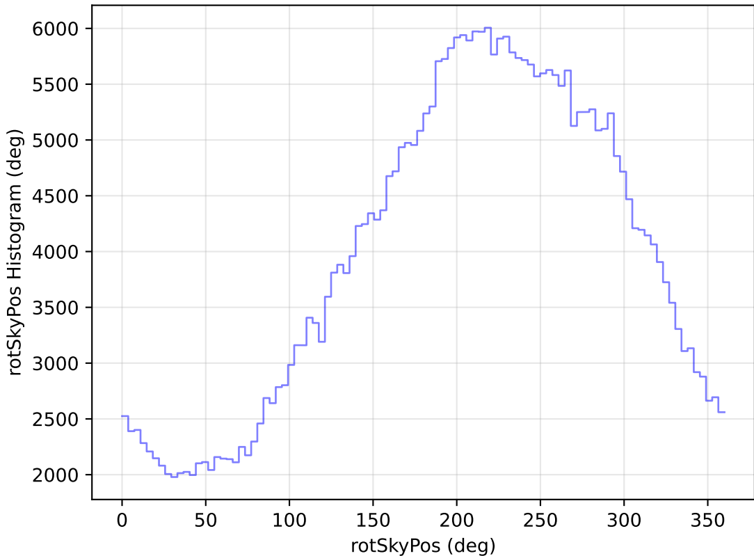
too_ignore_100_1v3.4_10yrs All sky y band: rotSkyPos Histogram
