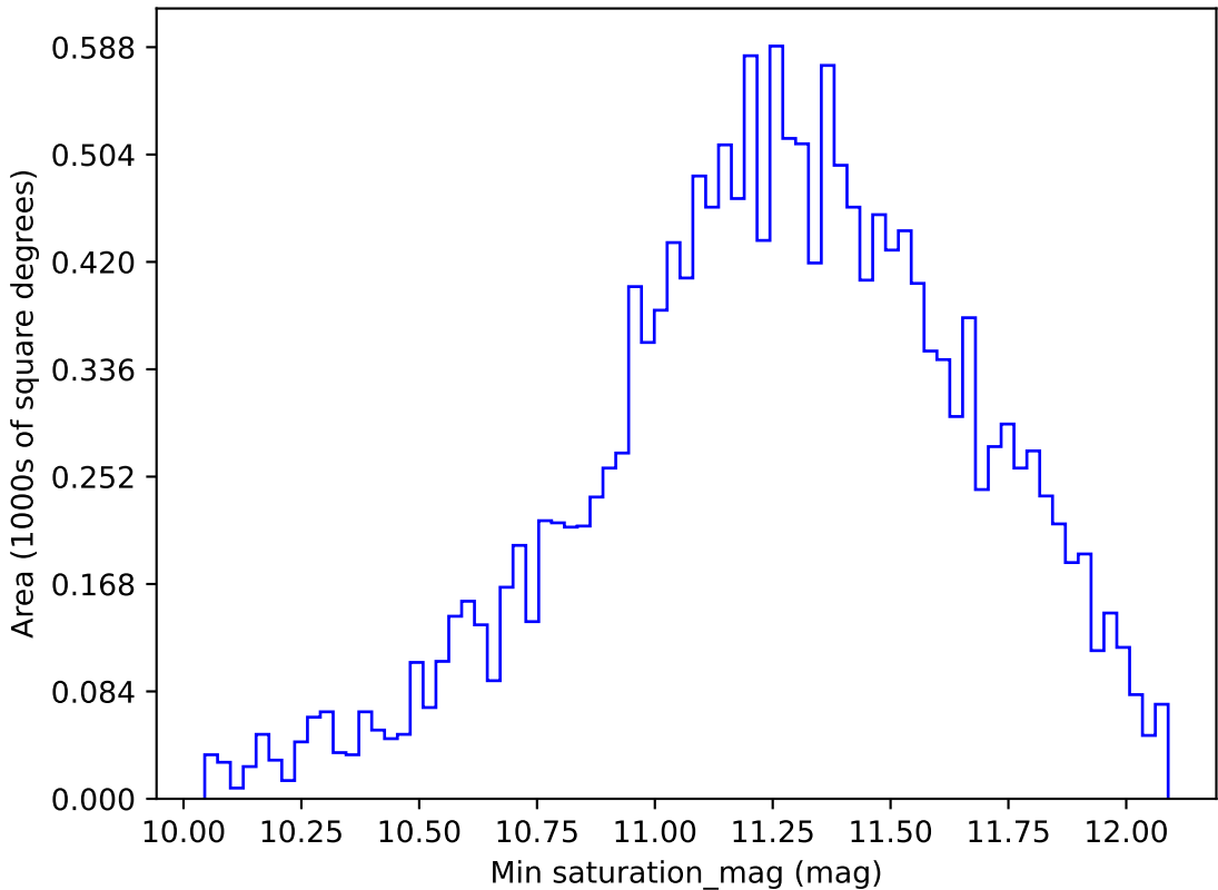
too_ignore_100_1v3.4_10yrs WFD y band: Min saturation_mag
