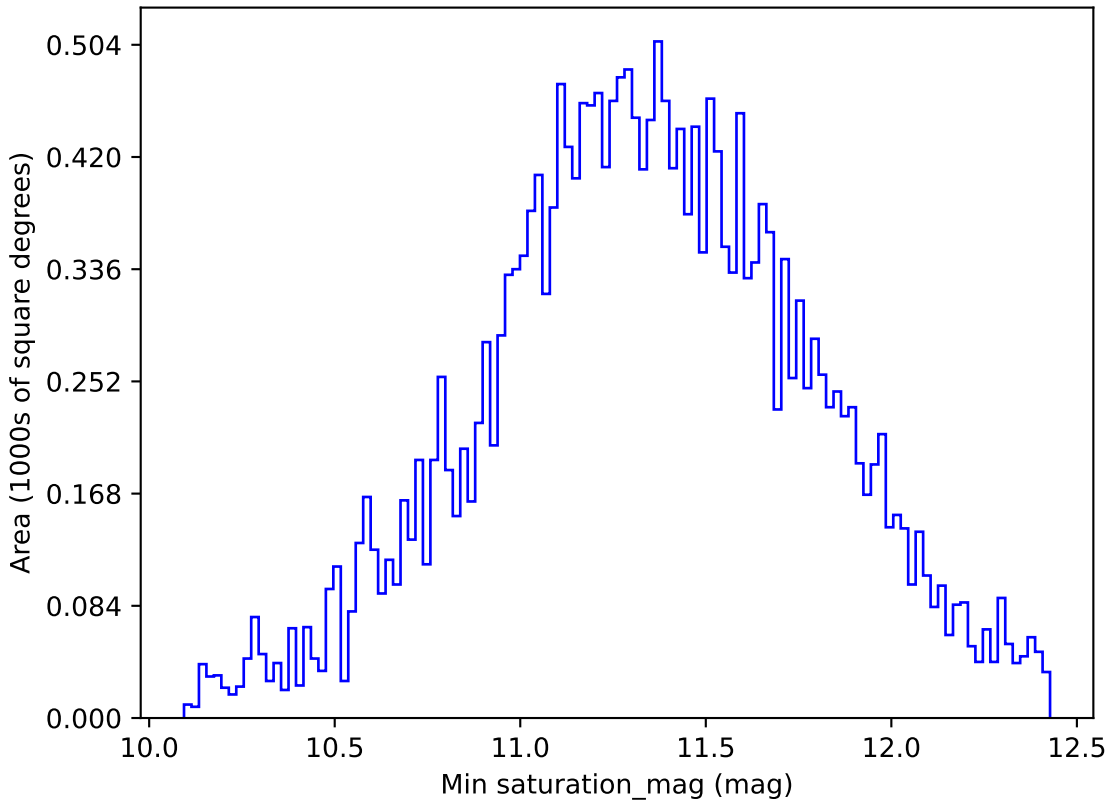
too_ignore_100_1v3.4_10yrs All sky y band: Min saturation_mag
