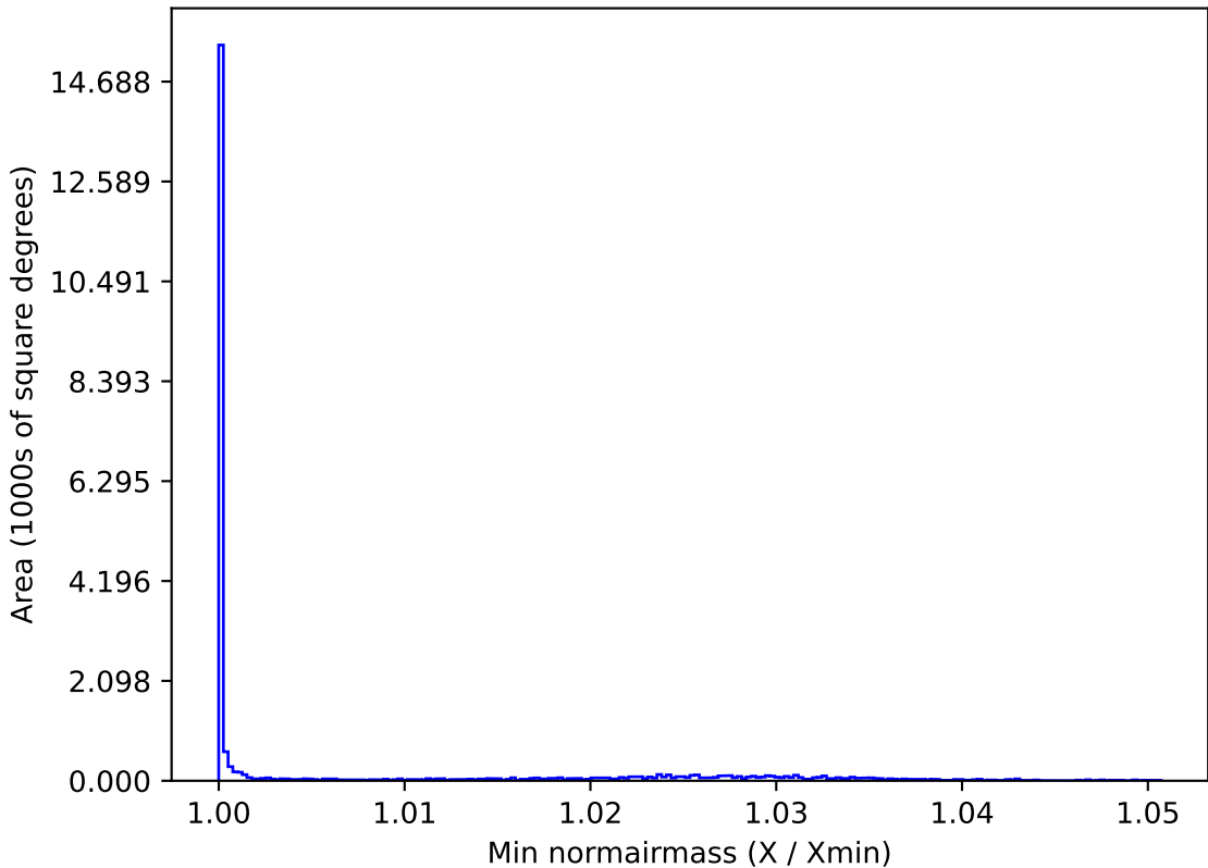
too_ignore_100_1v3.4_10yrs All sky y band: Min normairmass
