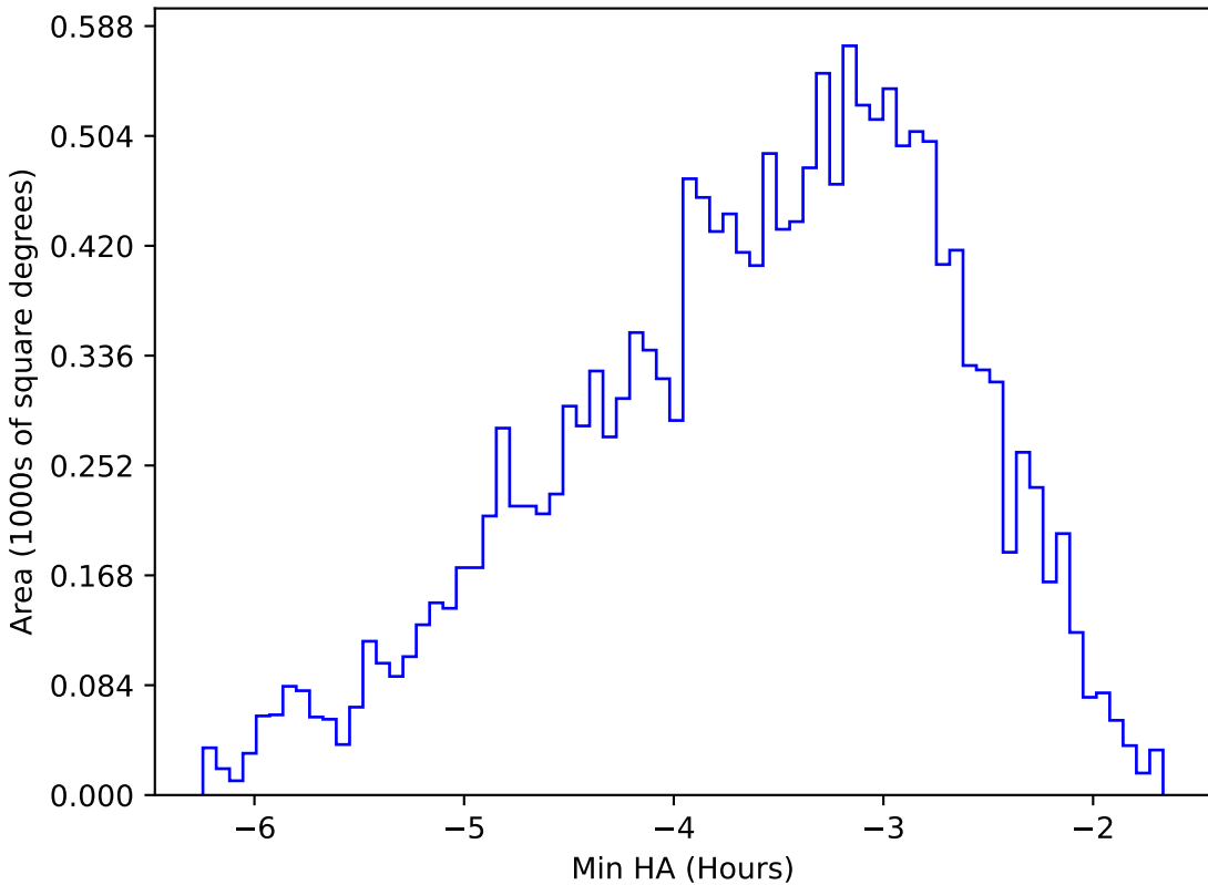
too_ignore_100_1v3.4_10yrs WFD y band: Min HA
