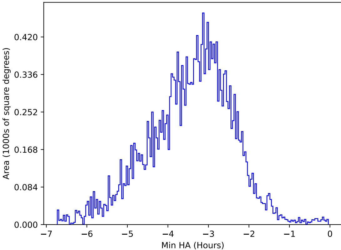
too_ignore_100_1v3.4_10yrs All sky y band: Min HA
