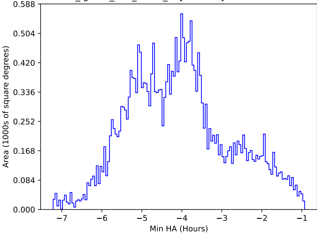
too_ignore_100_1v3.4_10yrs All sky i band: Min HA
