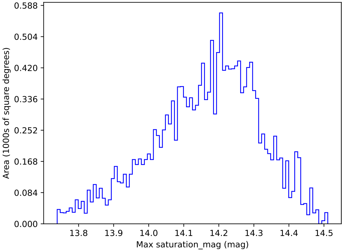
too_ignore_100_1v3.4_10yrs WFD y band: Max saturation_mag
