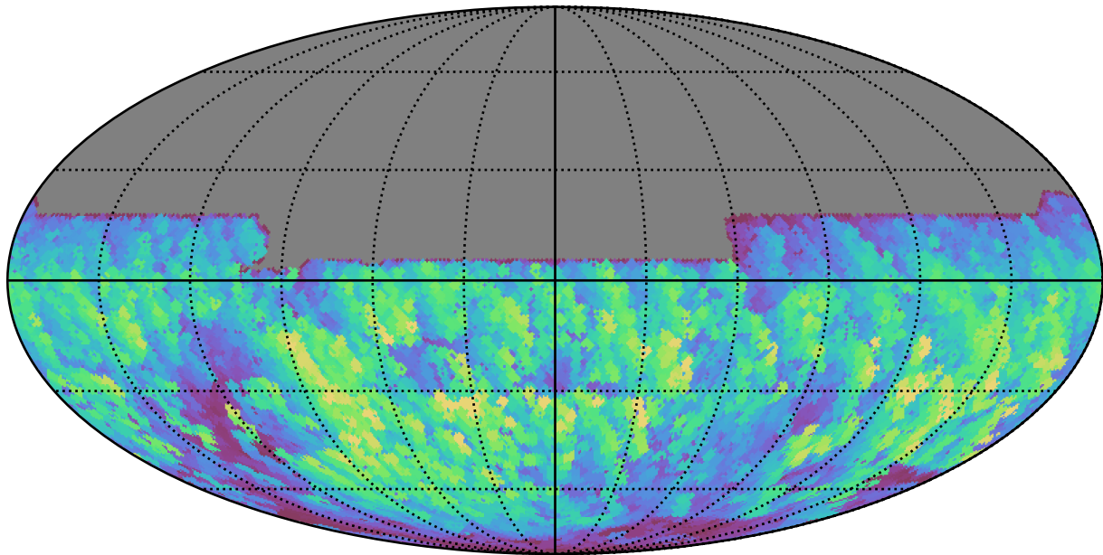
too_ignore_100_1v3.4_10yrs All sky y band: Max normairmass
