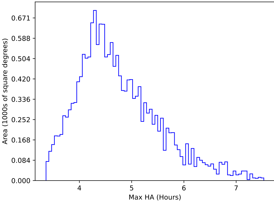
too_ignore_100_1v3.4_10yrs WFD y band: Max HA
