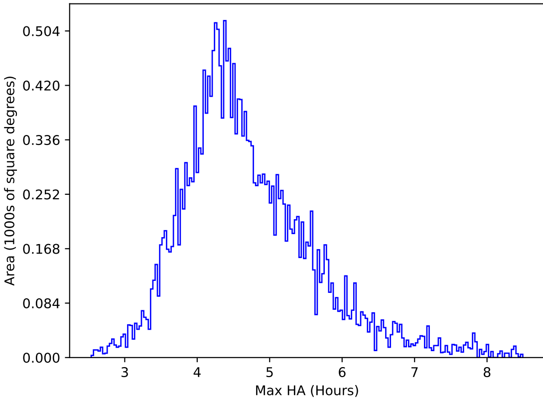
too_ignore_100_1v3.4_10yrs All sky y band: Max HA
