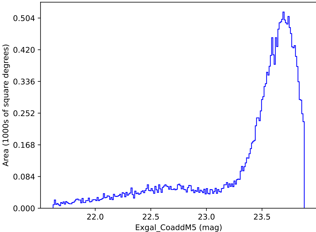
too_ignore_100_1v3.4_10yrs Yr 1 y band: Exgal_CoaddM5
