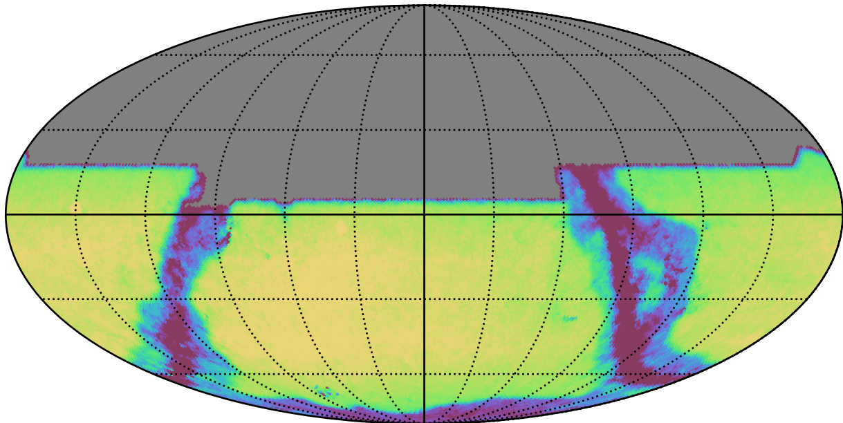
too_ignore_100_1v3.4_10yrs All sky y band: Exgal_CoaddM5
