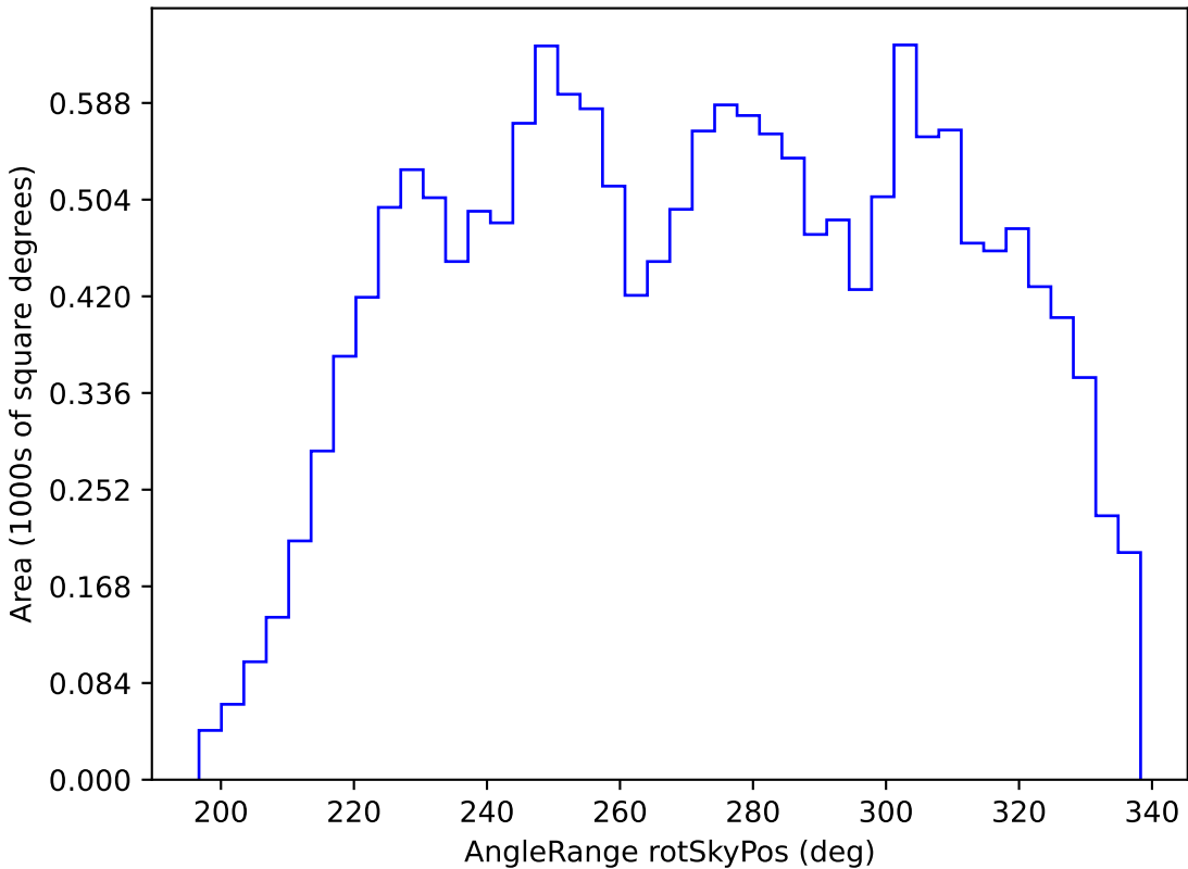
too_ignore_100_1v3.4_10yrs WFD y band: AngleRange rotSkyPos
