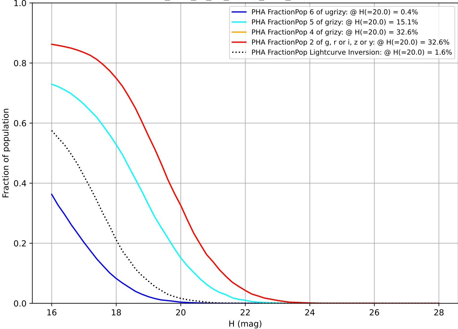
too_elab_r8_d3_ugrizy_v3.4_10yrs PHA
