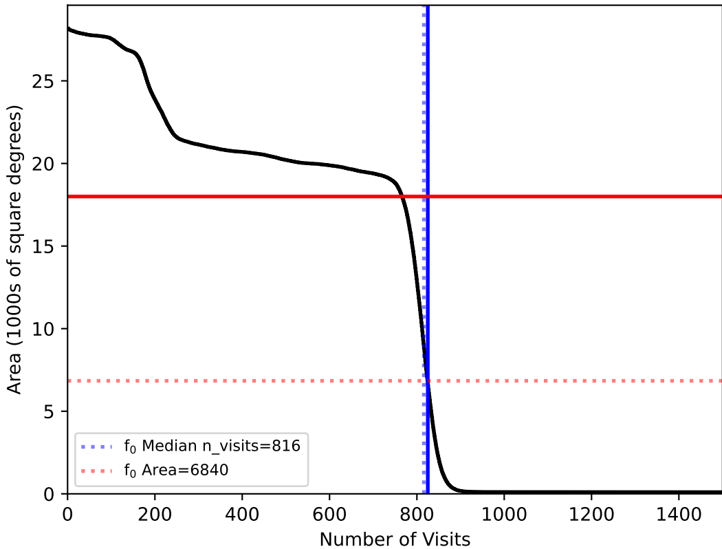
too_elab_r8_d3_ugrizy_v3.4_10yrs : fO
