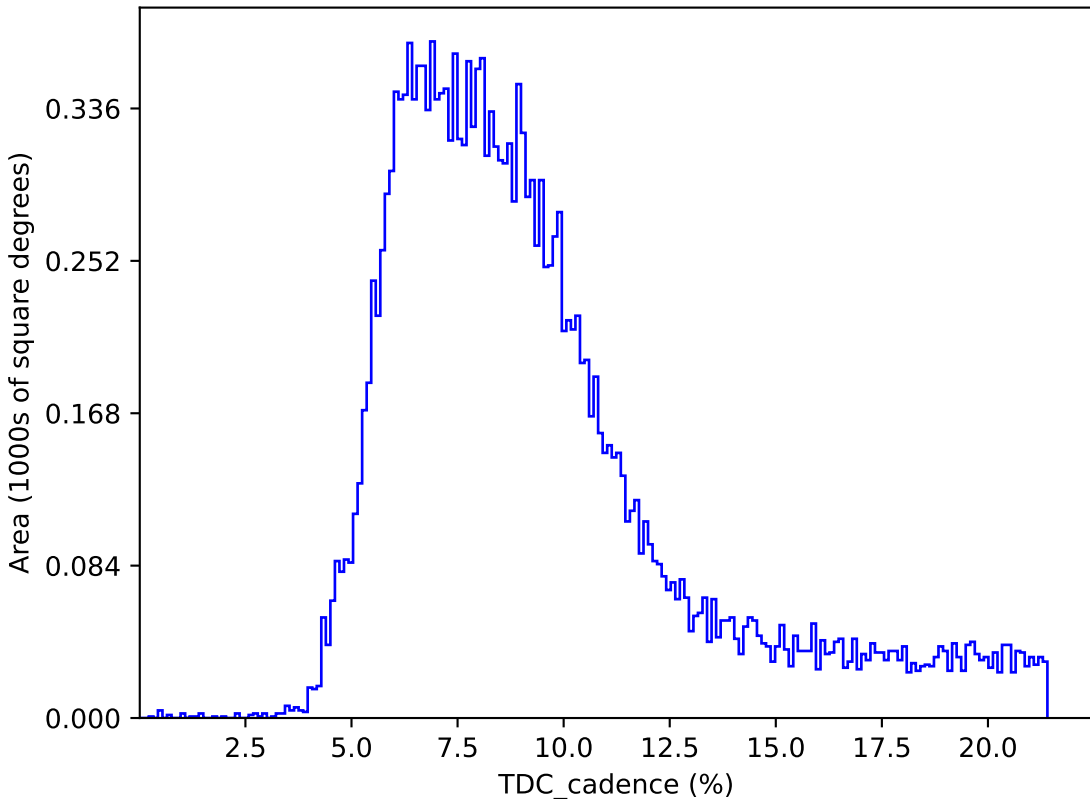
too_elab_r8_d3_ugrizy_v3.4_10yrs : TDC_cadence
