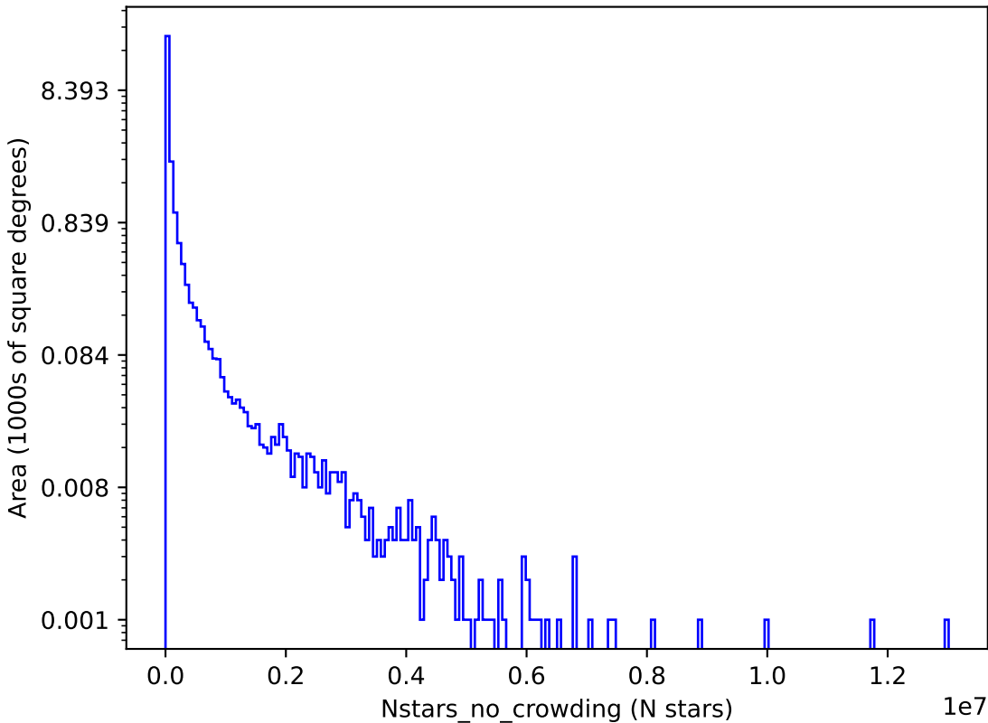
too_elab_r8_d3_ugrizy_v3.4_10yrs g: Nstars_no_crowding
