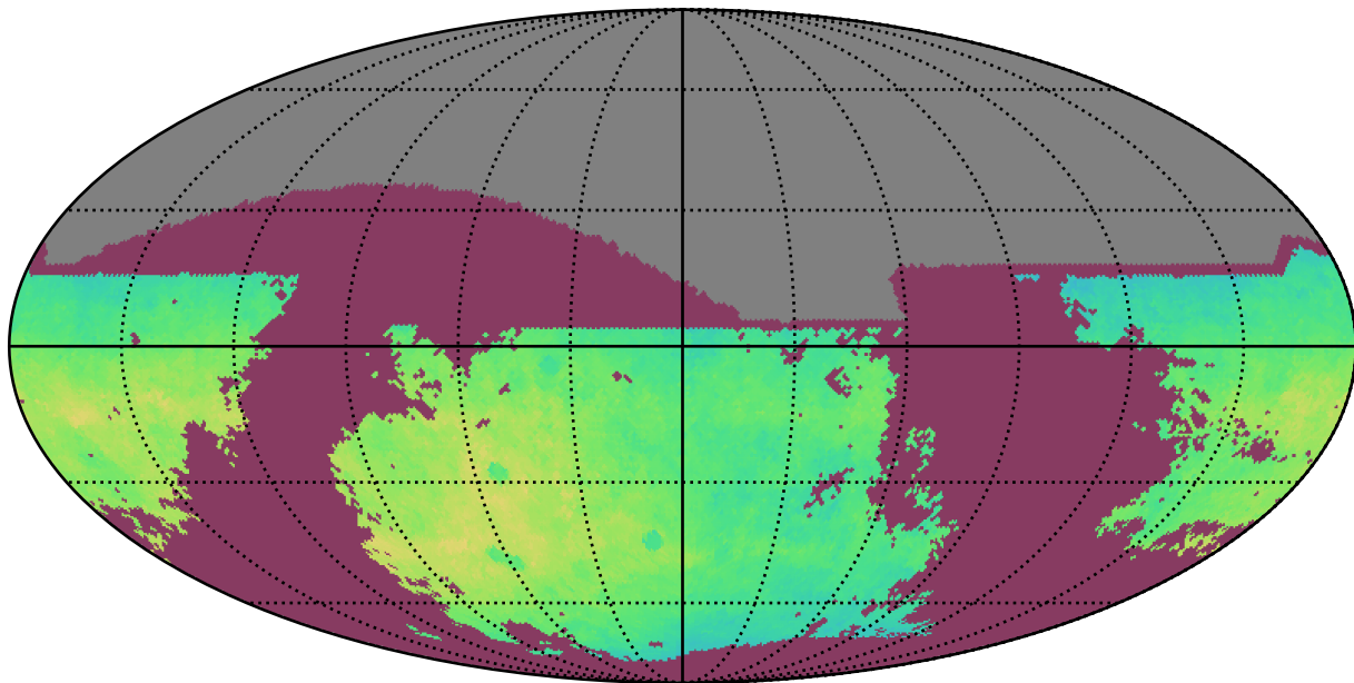
too_elab_r8_d3_ugrizy_v3.4_10yrs i: NgalScale
