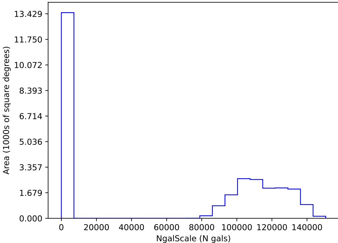
too_elab_r8_d3_ugrizy_v3.4_10yrs i: NgalScale
