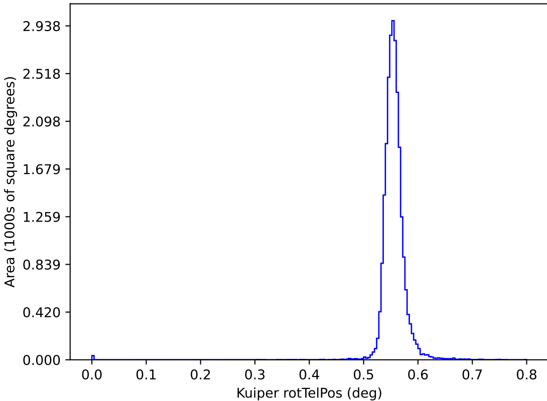
too_elab_r8_d3_ugrizy_v3.4_10yrs y: Kuiper rotTelPos
