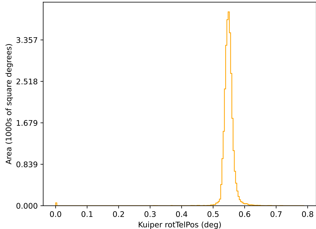
too_elab_r8_d3_ugrizy_v3.4_10yrs r: Kuiper rotTelPos
