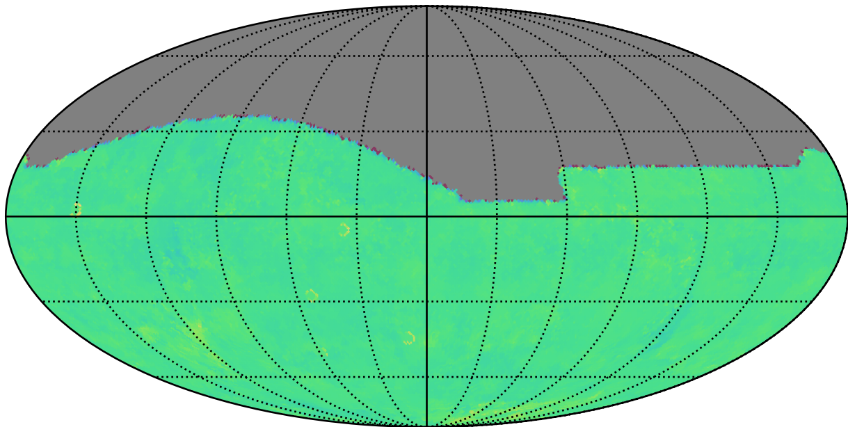
too_elab_r8_d3_ugrizy_v3.4_10yrs g: Kuiper rotTelPos
