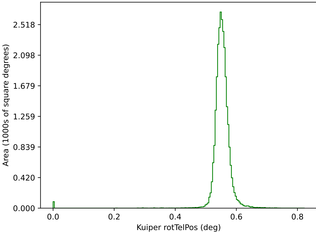
too_elab_r8_d3_ugrizy_v3.4_10yrs g: Kuiper rotTelPos
