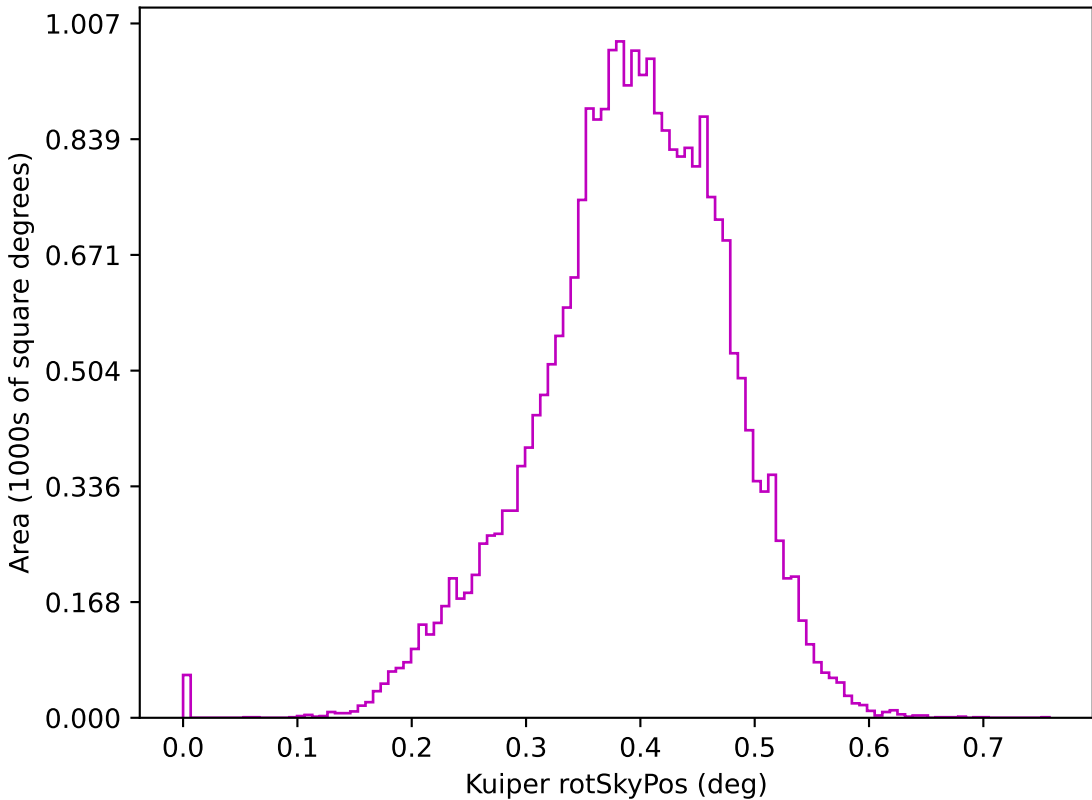
too_elab_r8_d3_ugrizy_v3.4_10yrs z: Kuiper rotSkyPos
