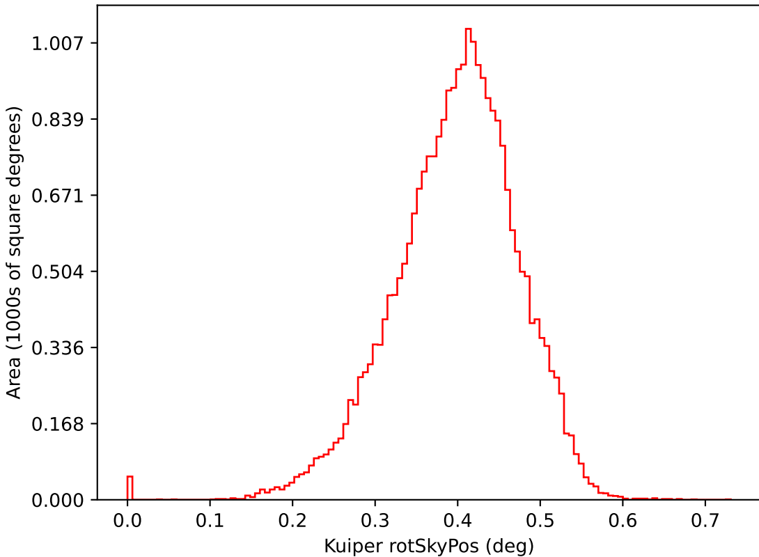
too_elab_r8_d3_ugrizy_v3.4_10yrs i: Kuiper rotSkyPos
