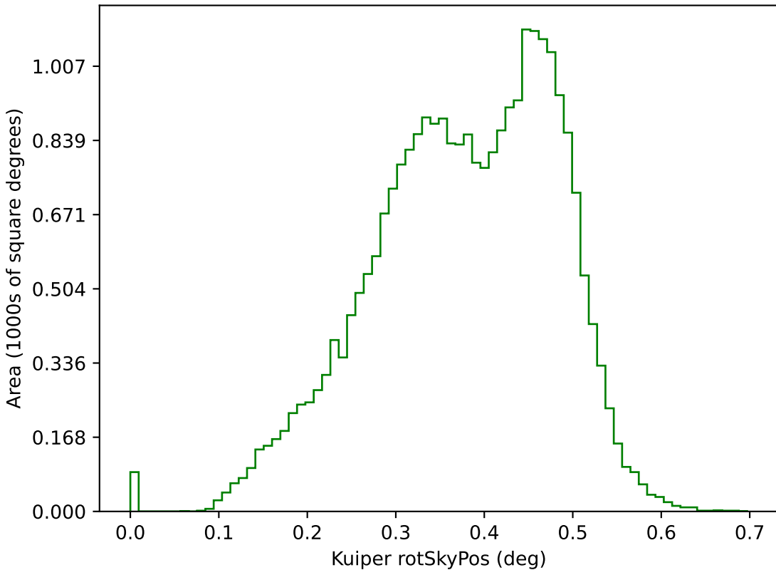
too_elab_r8_d3_ugrizy_v3.4_10yrs g: Kuiper rotSkyPos
