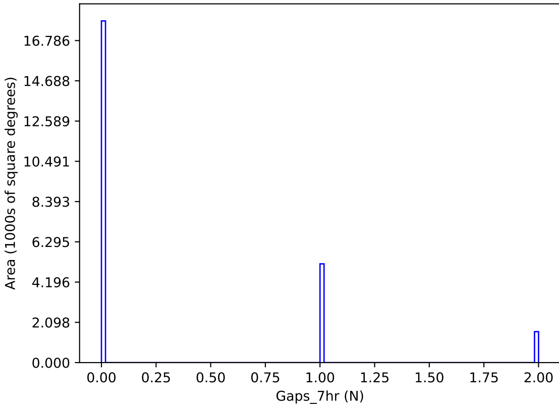
too_elab_r8_d3_ugrizy_v3.4_10yrs y band: Gaps_7hr
