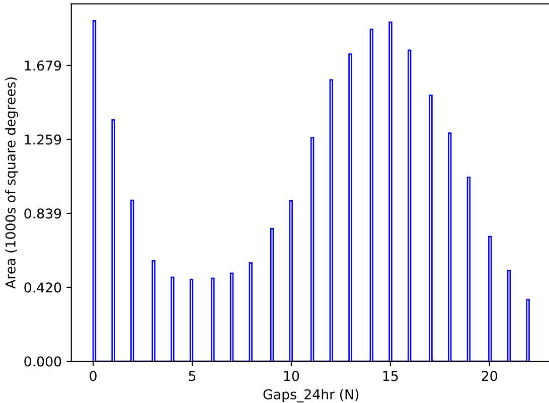
too_elab_r8_d3_ugrizy_v3.4_10yrs y band: Gaps_24hr
