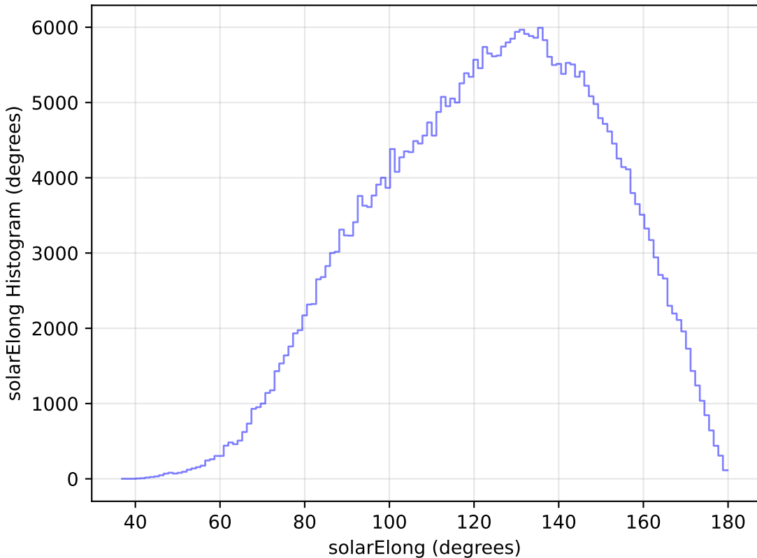
too_elab_r8_d3_ugrizy_v3.4_10yrs WFD y band: solarElong Histogram
