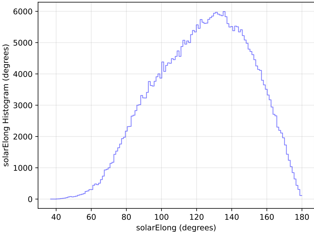
too_elab_r8_d3_ugrizy_v3.4_10yrs All sky y band: solarElong Histogram
