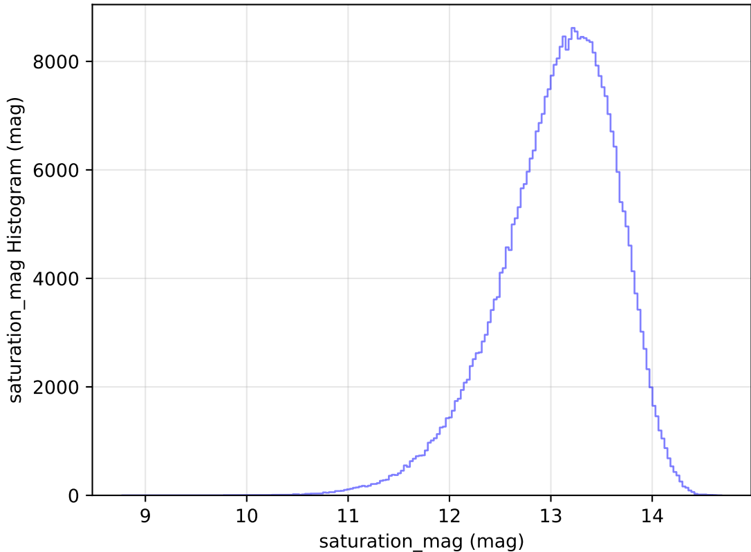
too_elab_r8_d3_ugrizy_v3.4_10yrs All sky y band: saturation_mag Histogram
