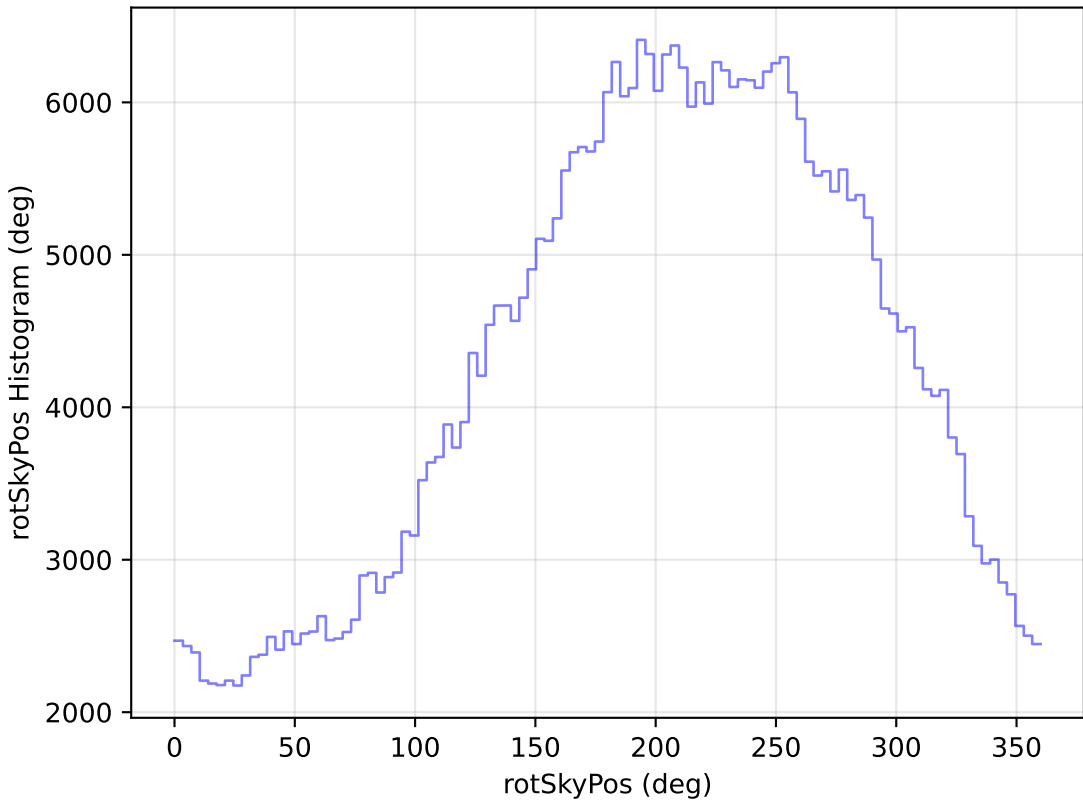
too_elab_r8_d3_ugrizy_v3.4_10yrs WFD z band: rotSkyPos Histogram
