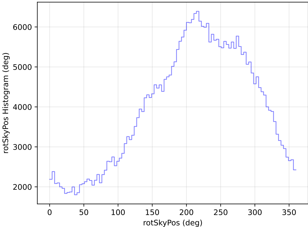
too_elab_r8_d3_ugrizy_v3.4_10yrs WFD y band: rotSkyPos Histogram
