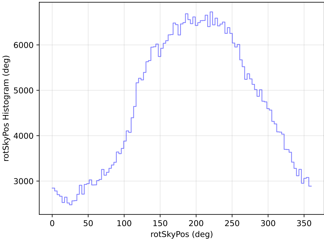
too_elab_r8_d3_ugrizy_v3.4_10yrs WFD r band: rotSkyPos Histogram
