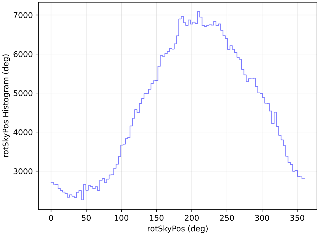
too_elab_r8_d3_ugrizy_v3.4_10yrs WFD i band: rotSkyPos Histogram
