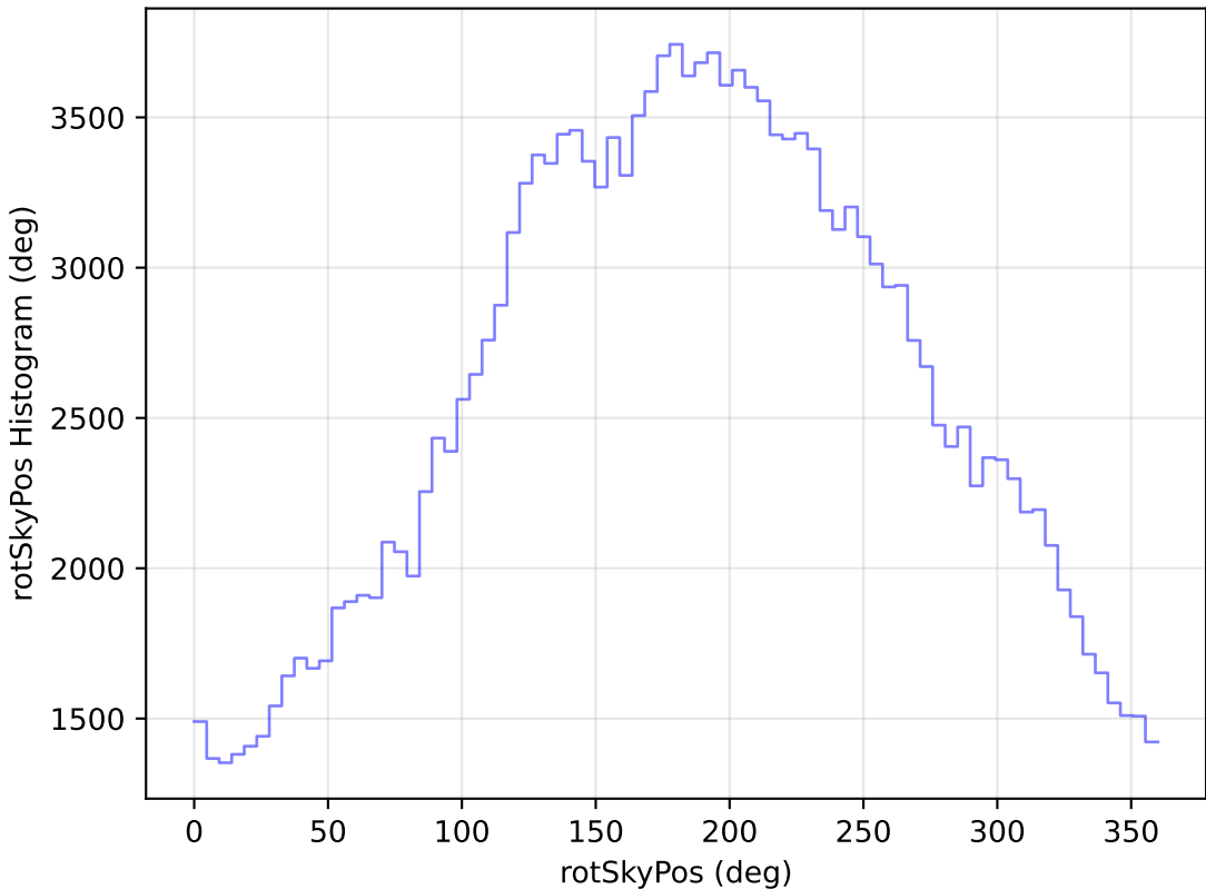
too_elab_r8_d3_ugrizy_v3.4_10yrs WFD g band: rotSkyPos Histogram
