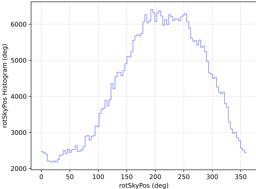
too_elab_r8_d3_ugrizy_v3.4_10yrs All sky z band: rotSkyPos Histogram
