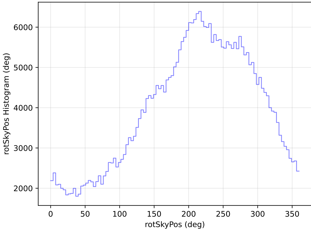
too_elab_r8_d3_ugrizy_v3.4_10yrs All sky y band: rotSkyPos Histogram
