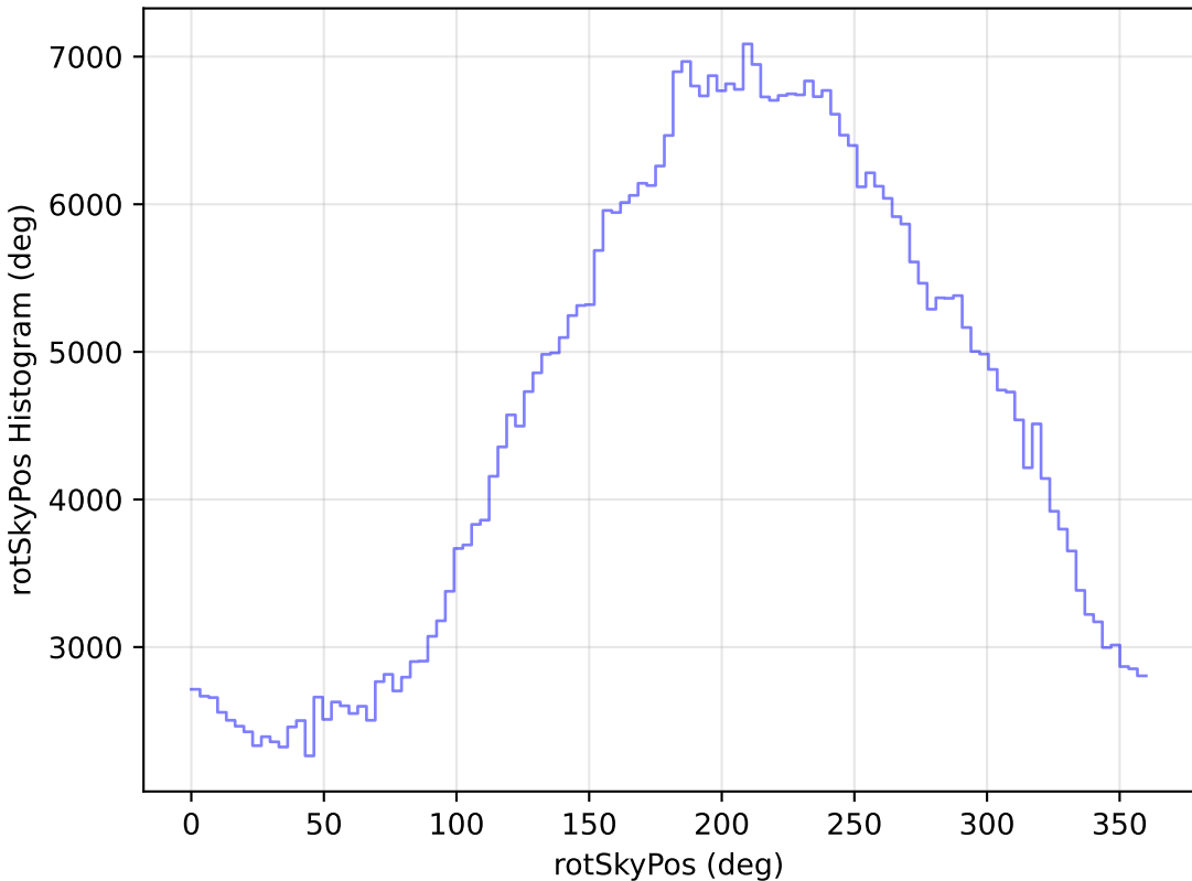
too_elab_r8_d3_ugrizy_v3.4_10yrs All sky i band: rotSkyPos Histogram
