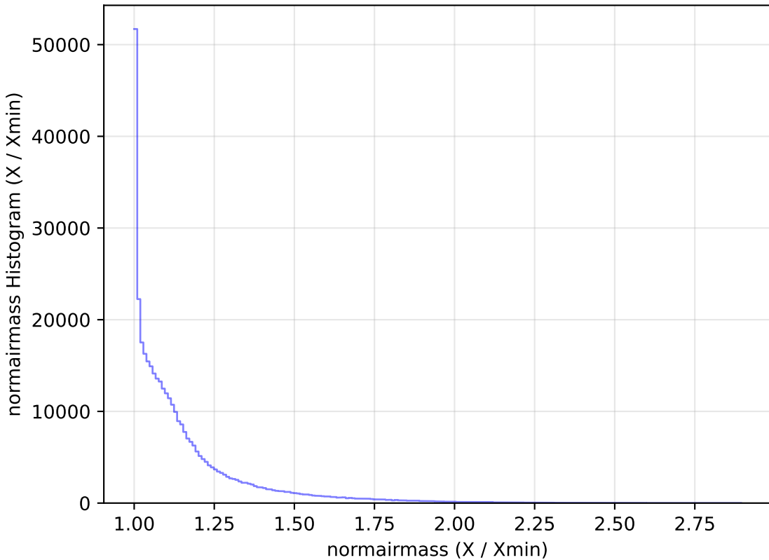
too_elab_r8_d3_ugrizy_v3.4_10yrs WFD y band: normairmass Histogram
