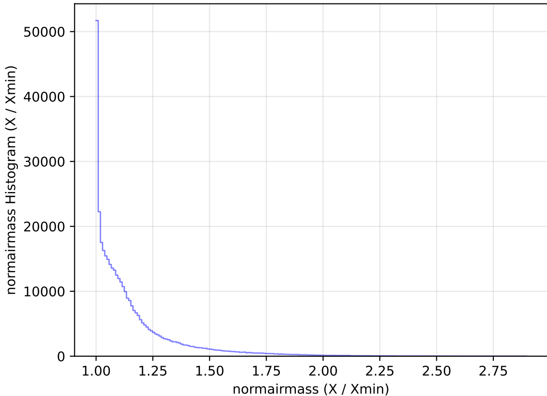
too_elab_r8_d3_ugrizy_v3.4_10yrs All sky y band: normairmass Histogram
