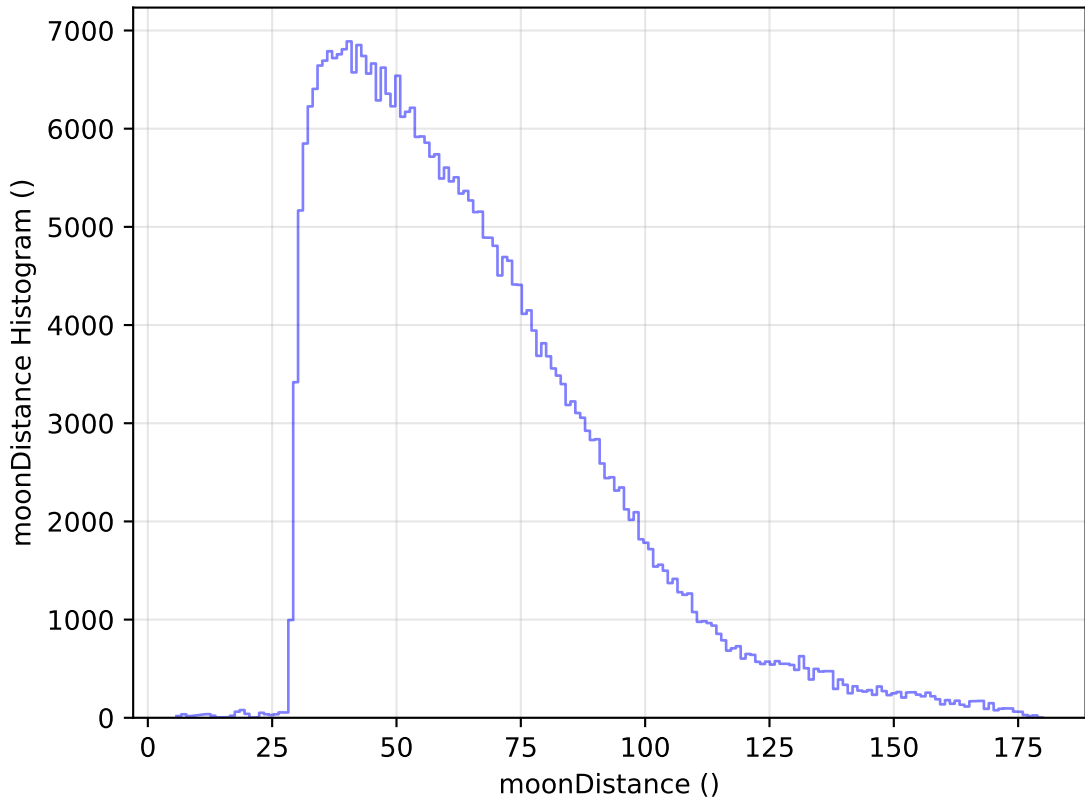
too_elab_r8_d3_ugrizy_v3.4_10yrs WFD y band: moonDistance Histogram
