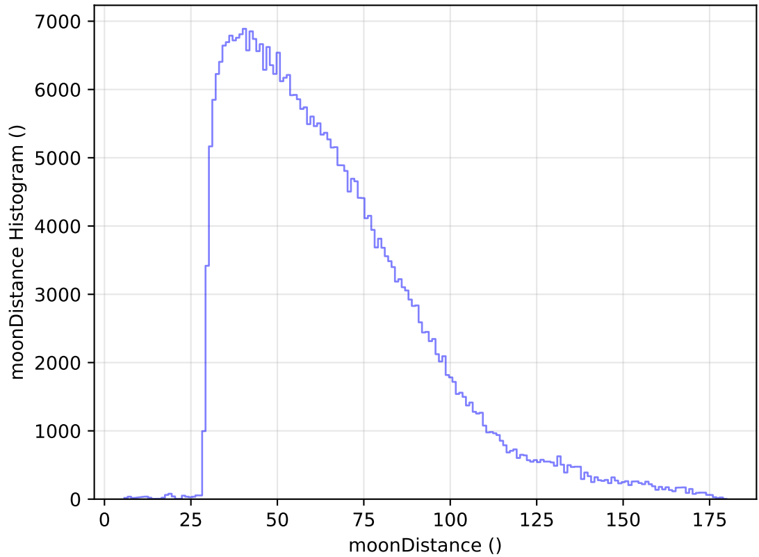
too_elab_r8_d3_ugrizy_v3.4_10yrs All sky y band: moonDistance Histogram
