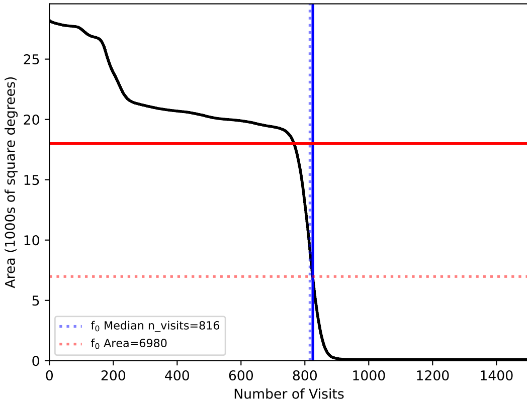
too_elab_r8_d3_ugrizy_v3.4_10yrs All sky: f0
