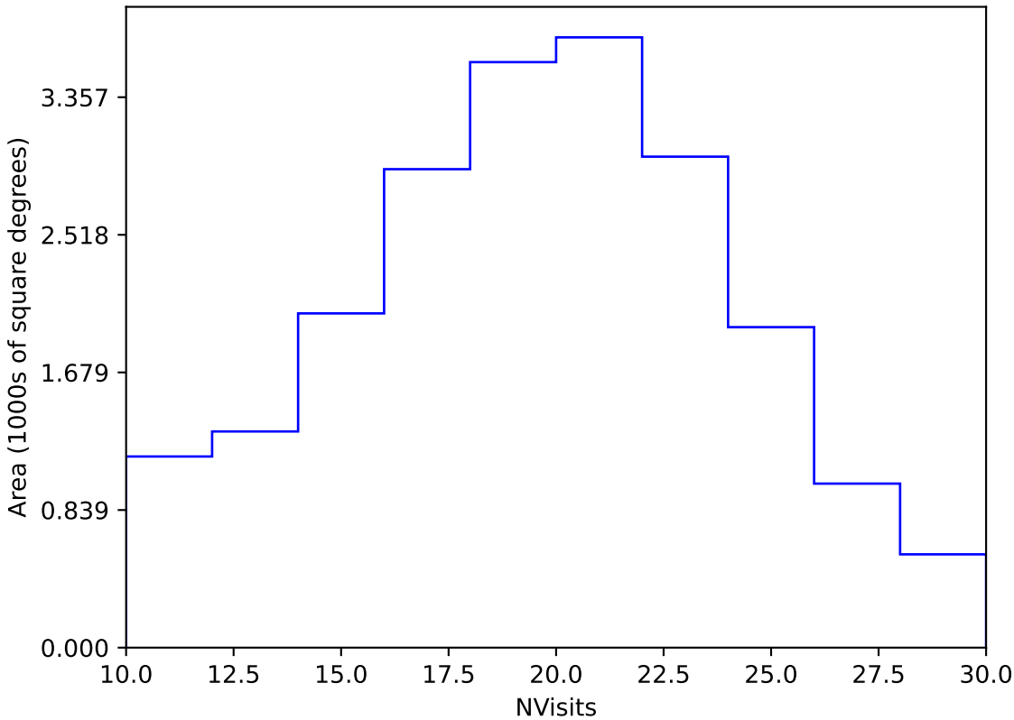
too_elab_r8_d3_ugrizy_v3.4_10yrs Yr 1 y band: NVisits
